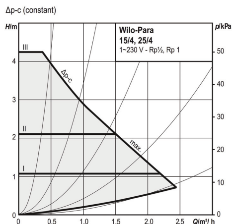
Kennlinien Wilo-Para, konstanter Differenzdruck
